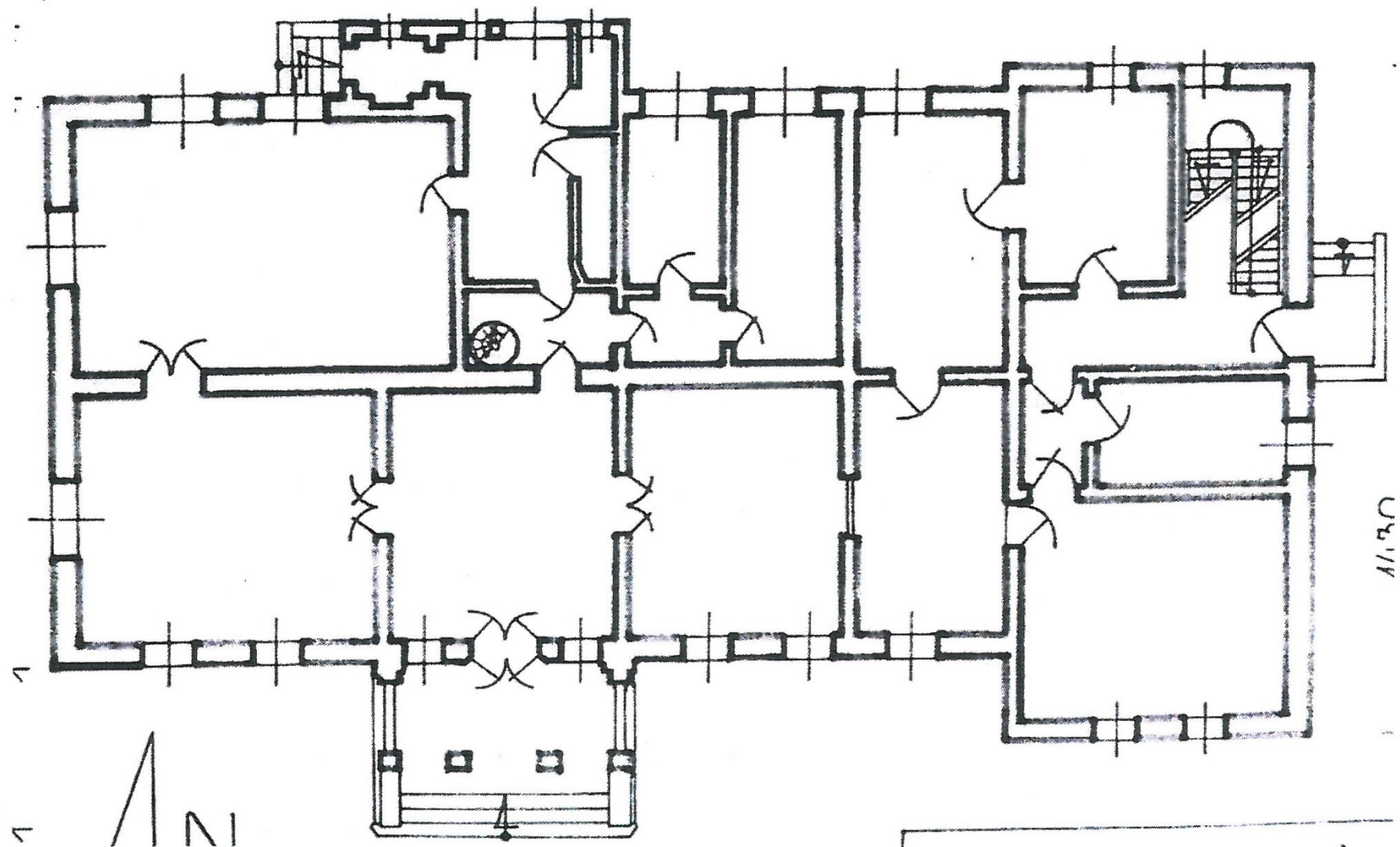
Dwór w Bagdadzie. Plan parteru
